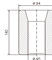
滤芯尺寸
