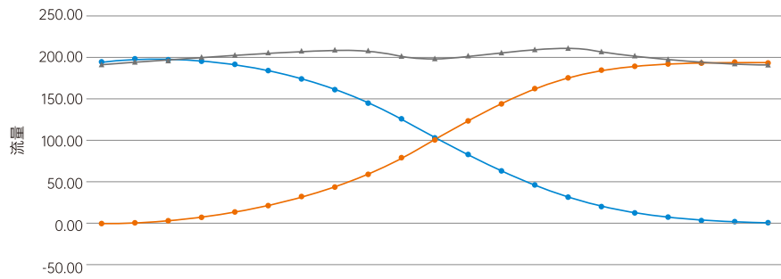
三花 EBV-309 三通电动球阀 流量曲线与脉冲数关系
